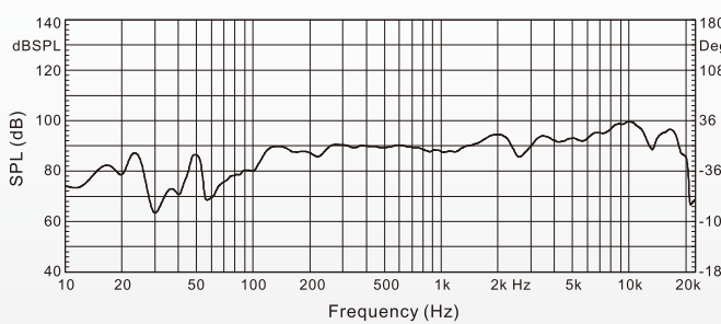
CMX6903 频率响应曲线
