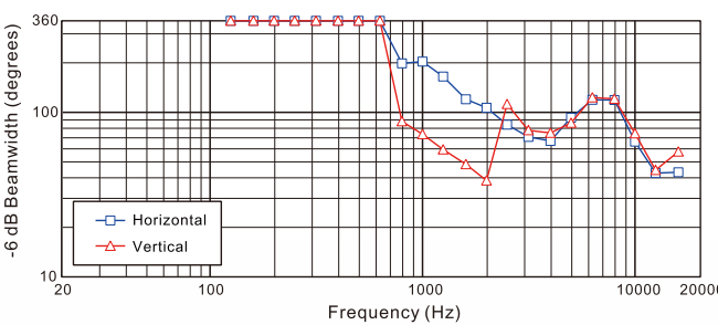
CMX6403 覆盖范围曲线
