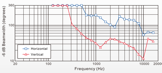
CMX6903 覆盖范围曲线
