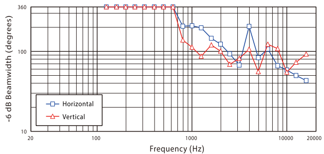
CMX6203 覆盖范围曲线
