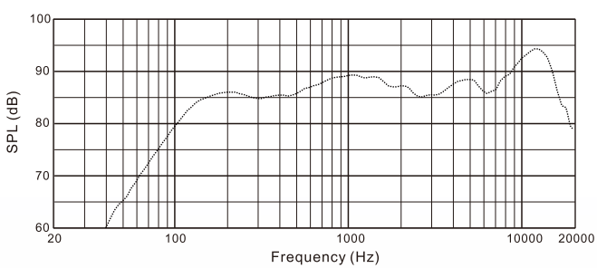
CMX6403 频率响应曲线
